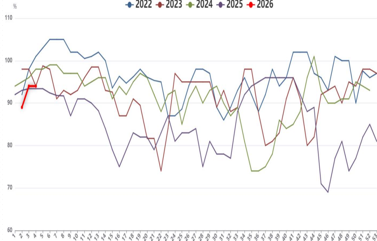
辛醇开工率
