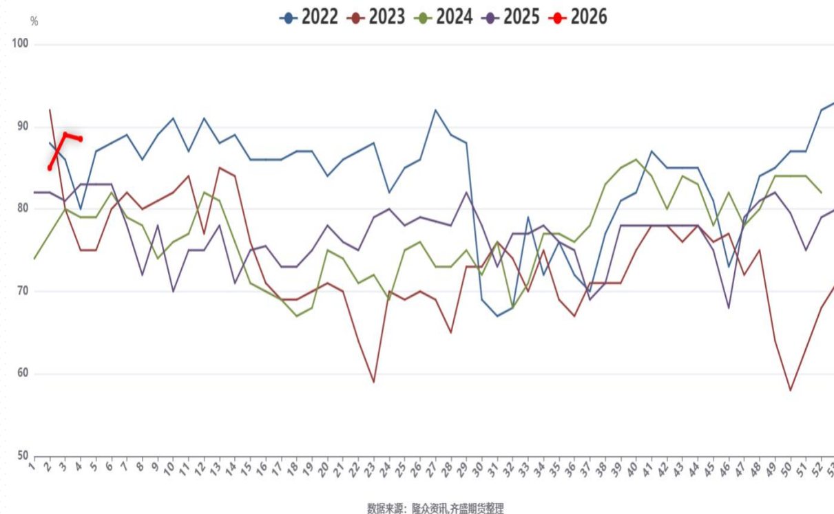
酚酮开工率
