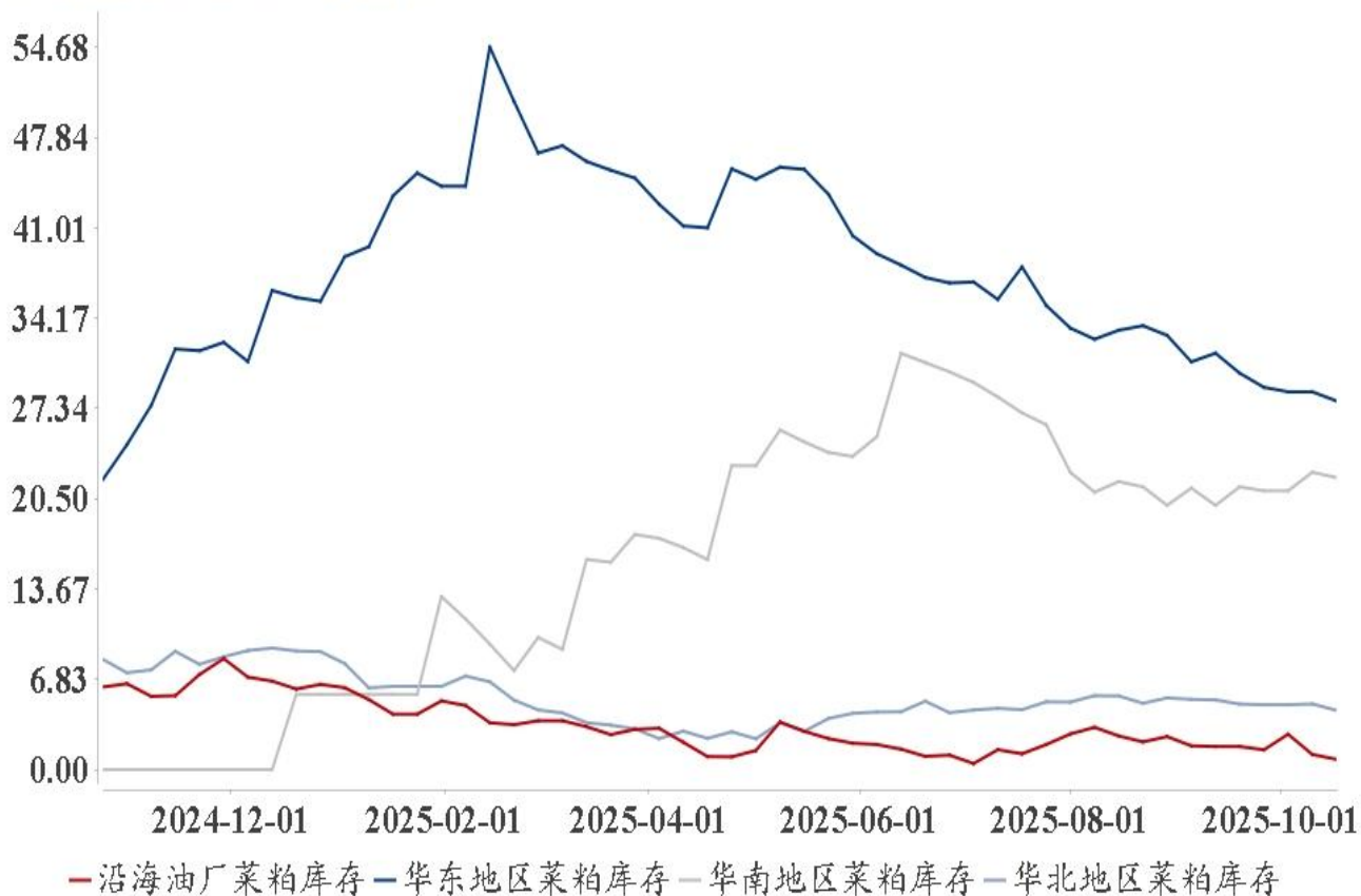
全国主要地区菜粕库存走势图
